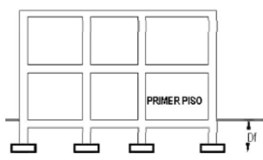
PROFUNDIDAD DE CIMENTACION ( D_f ) EN ZAPATAS SUPERFICIALES
